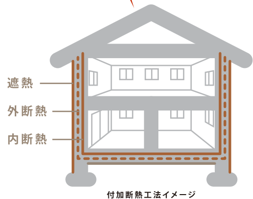
付加断熱工法イメージ
